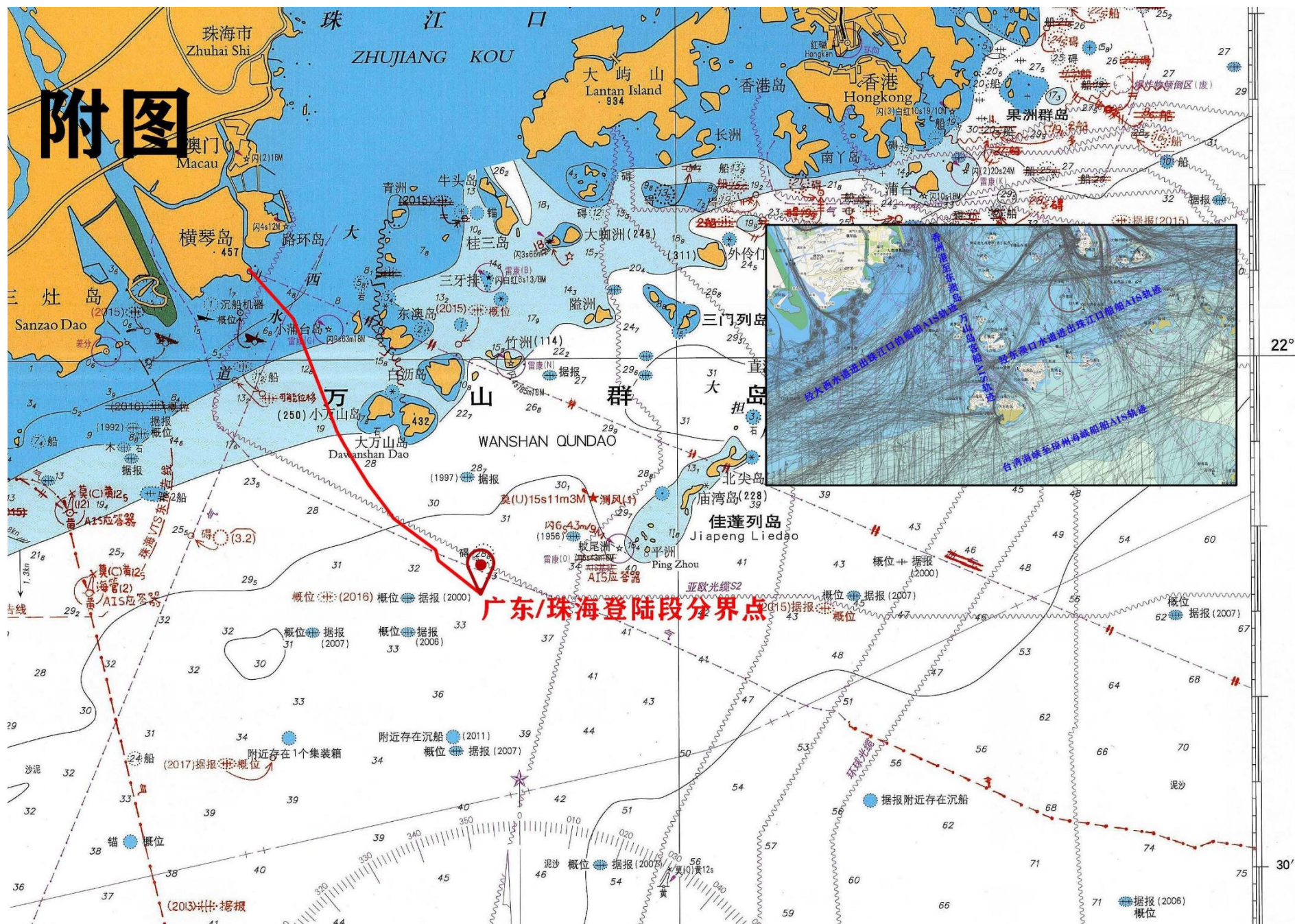
添付 1. 海底ケーブル経路略図
